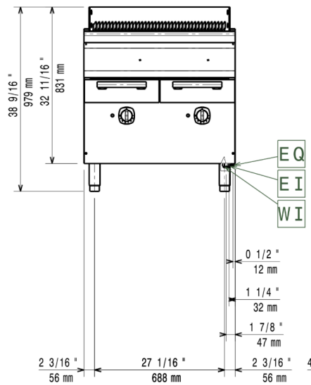
Edestä
