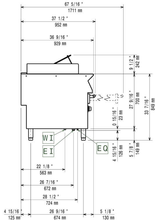
Sivulta
